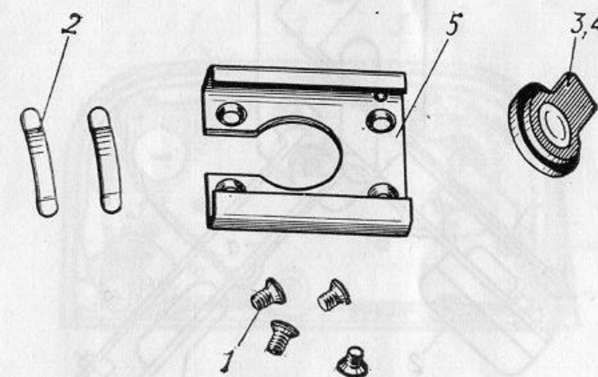
Рис. 23. Обойма (бескабельной лампы-вспышки):
