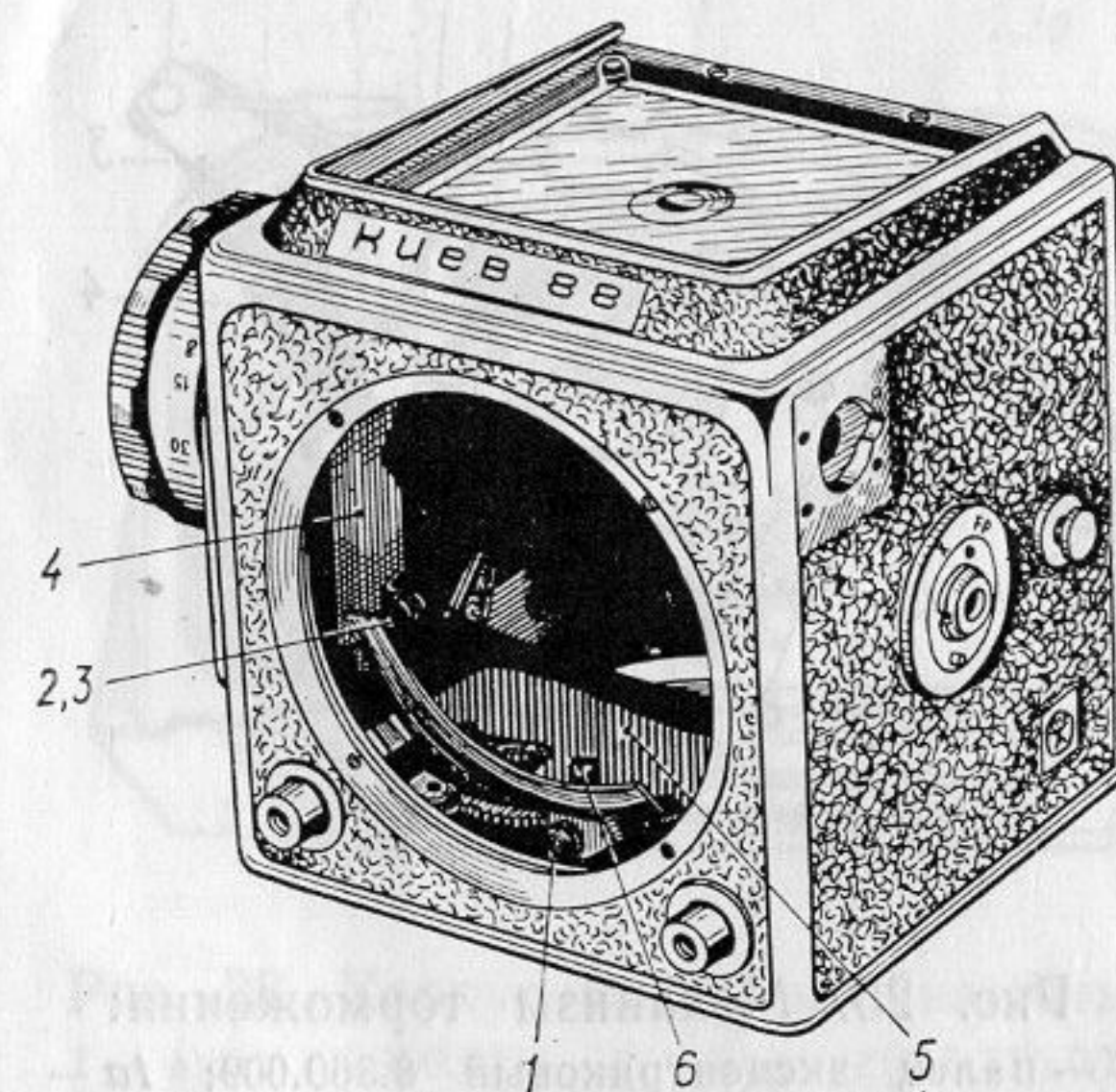
Рис. 20. Фотокамера (вид четвертый):
