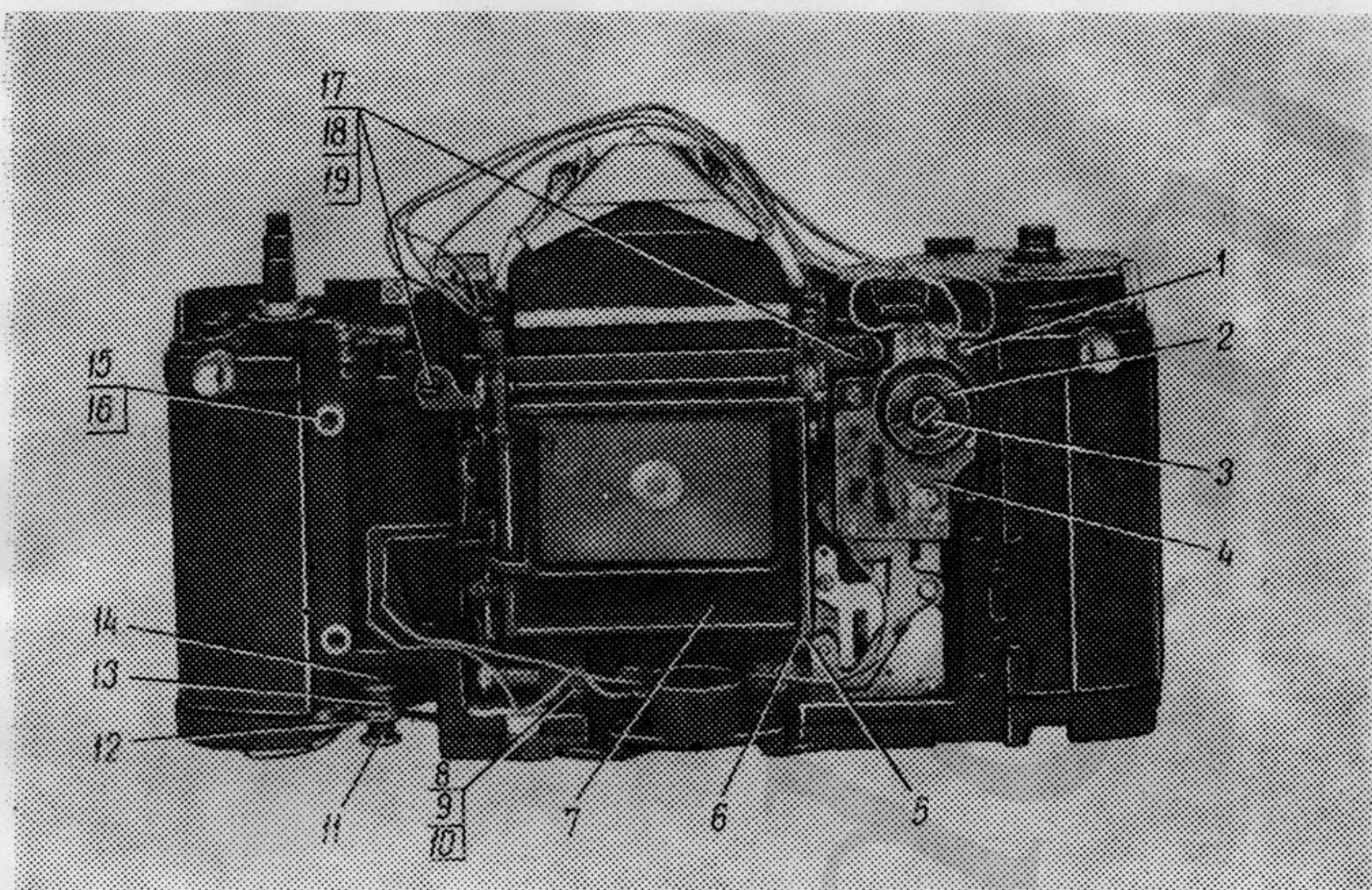
1—винт 8.900.422; 2—втулка 9.120.674; 3—винт 8.900.029; 4—механизм ввода выдержек 5.822.185; 5—рычаг 8.332.495; 6—рычаг 6.354.679; 7—зеркало 5.950.503; 8—винт 8.909.430; 9—шайба 8.942.042; 10—шайба 8.942.535; 11—винт 8.900.006; 12—гайка 8.934.948; 13—пружина 8.383.616; 14—фрикцион 5.822.100; 15—шайба 8.942.042; 16—шайба 8.942.535; 17—винт 8.909.699; 18—шайба 8.942.042; 19—шайба 8.942.535
