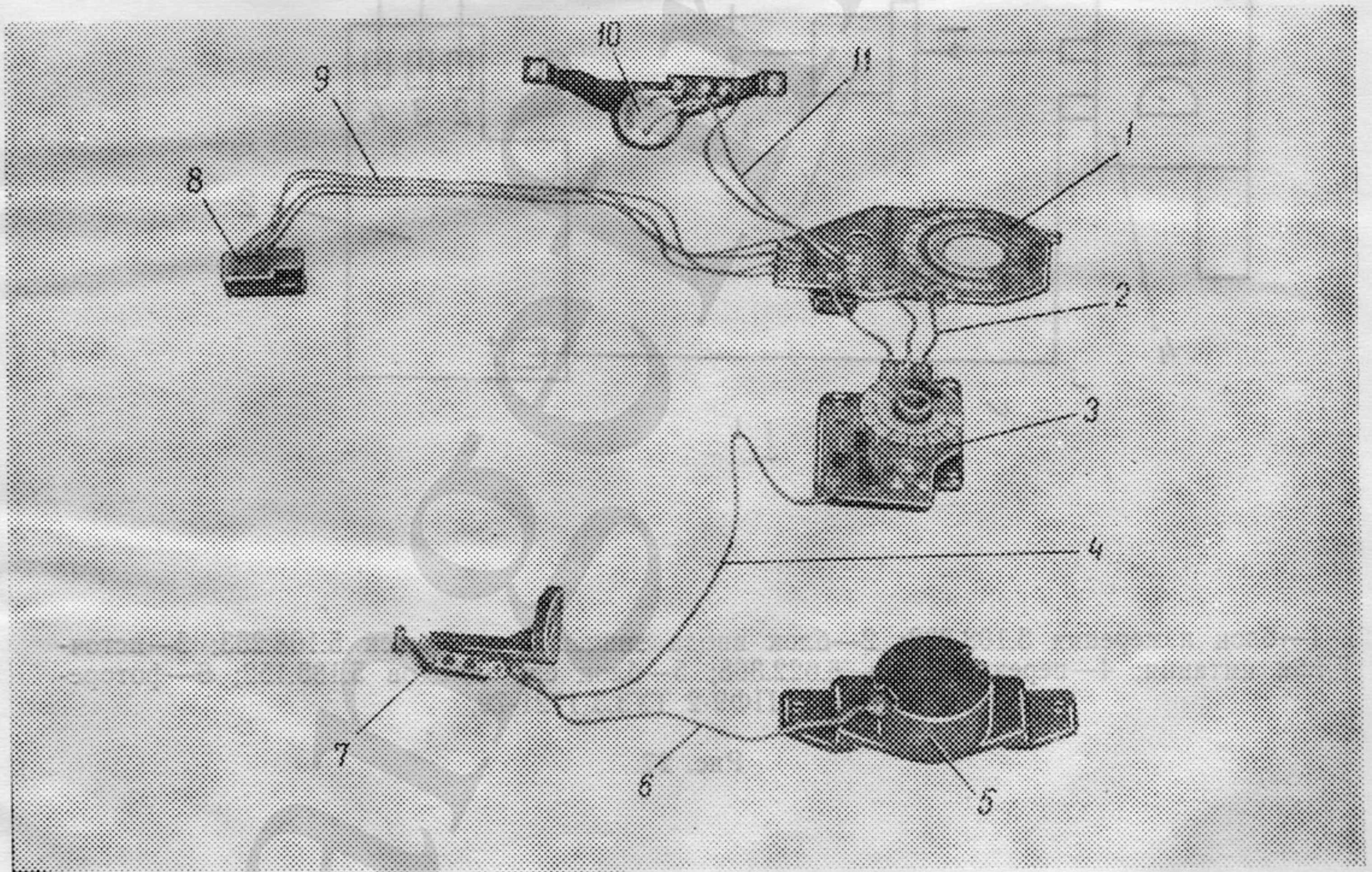
1—микросборка 5.108.232; 2—провод 7.760.132-01/02; 3—микросборка 5.108.233; 4—провод 7.760.132-14; 5—корпус 6.675.118; 6—провод 7.760.132-10; 7—контакт 6.622.368; 8—блок светодиодов 5.185.152; 9—провод 7.760.132-14; 10—фоторезистор 5.641.039; 11—провод 7.760.132-08.
