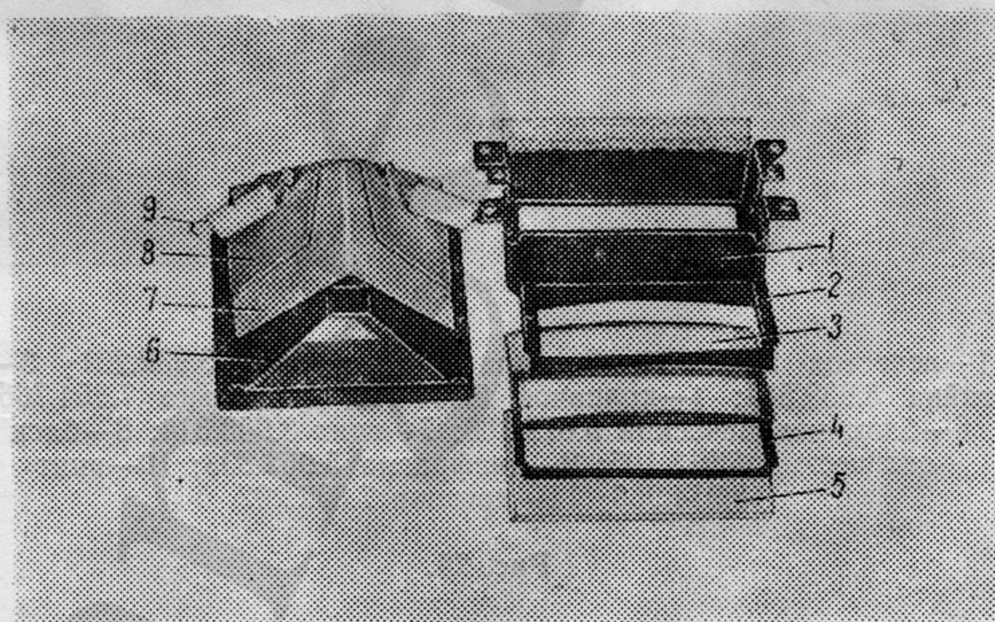
1—корпус 6.118.065; 2—прокладка 8.603.700; 3—линза 7.526.065; 4—прокладка 8.685.539; 5—линза Френеля 7.249.105; 6—призма 7.201.184; 7—прокладка 8.685.541; 8—накладка 8.604.616; 9—пружина 8.389.105.
