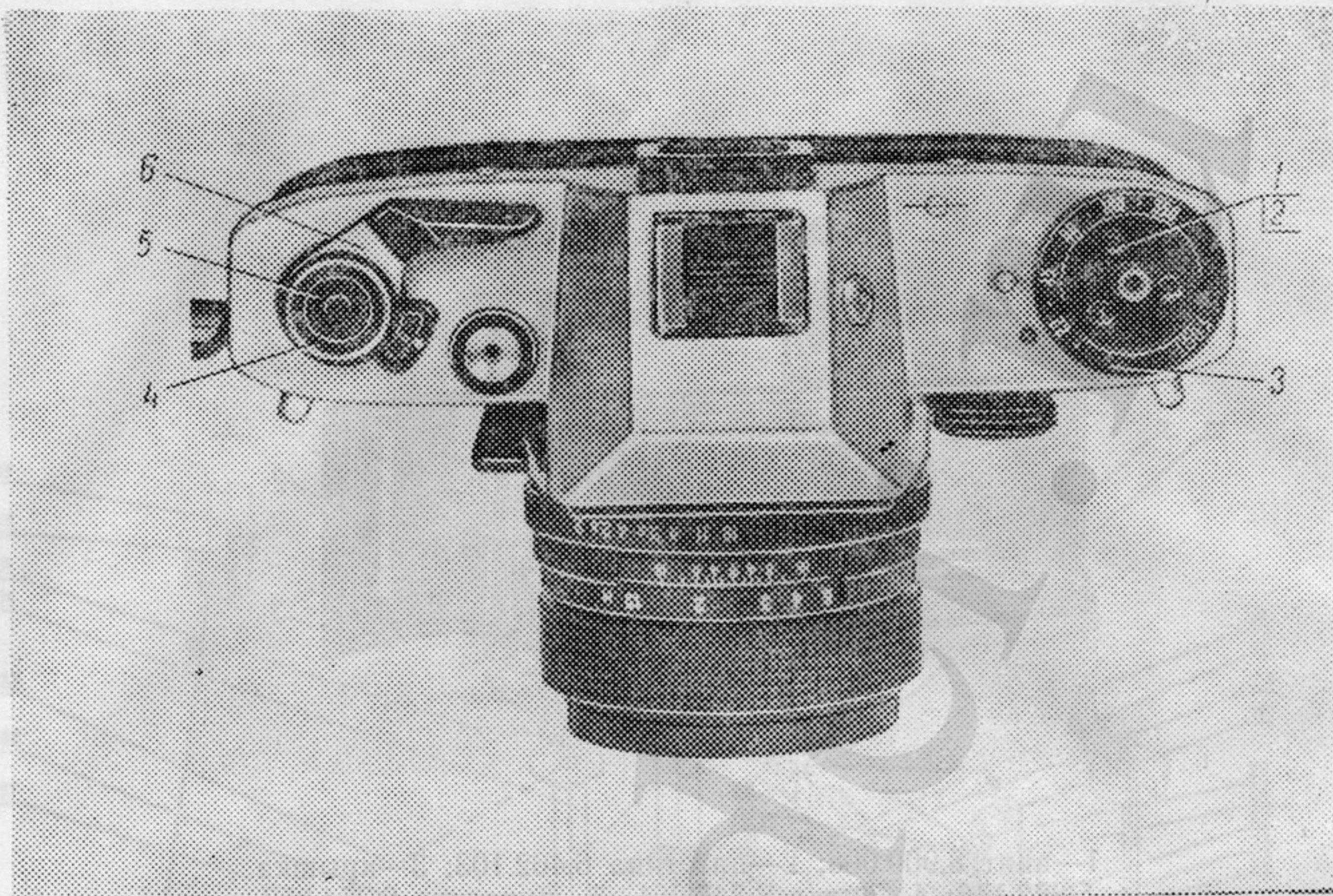
1—винт 8.903.034; 2—шайба 8.942.072; 3—шкала 7.021.502; 4—втулка 8.229.519; 5—гайка 9.438.253; 6—рычаг 6.354.480
