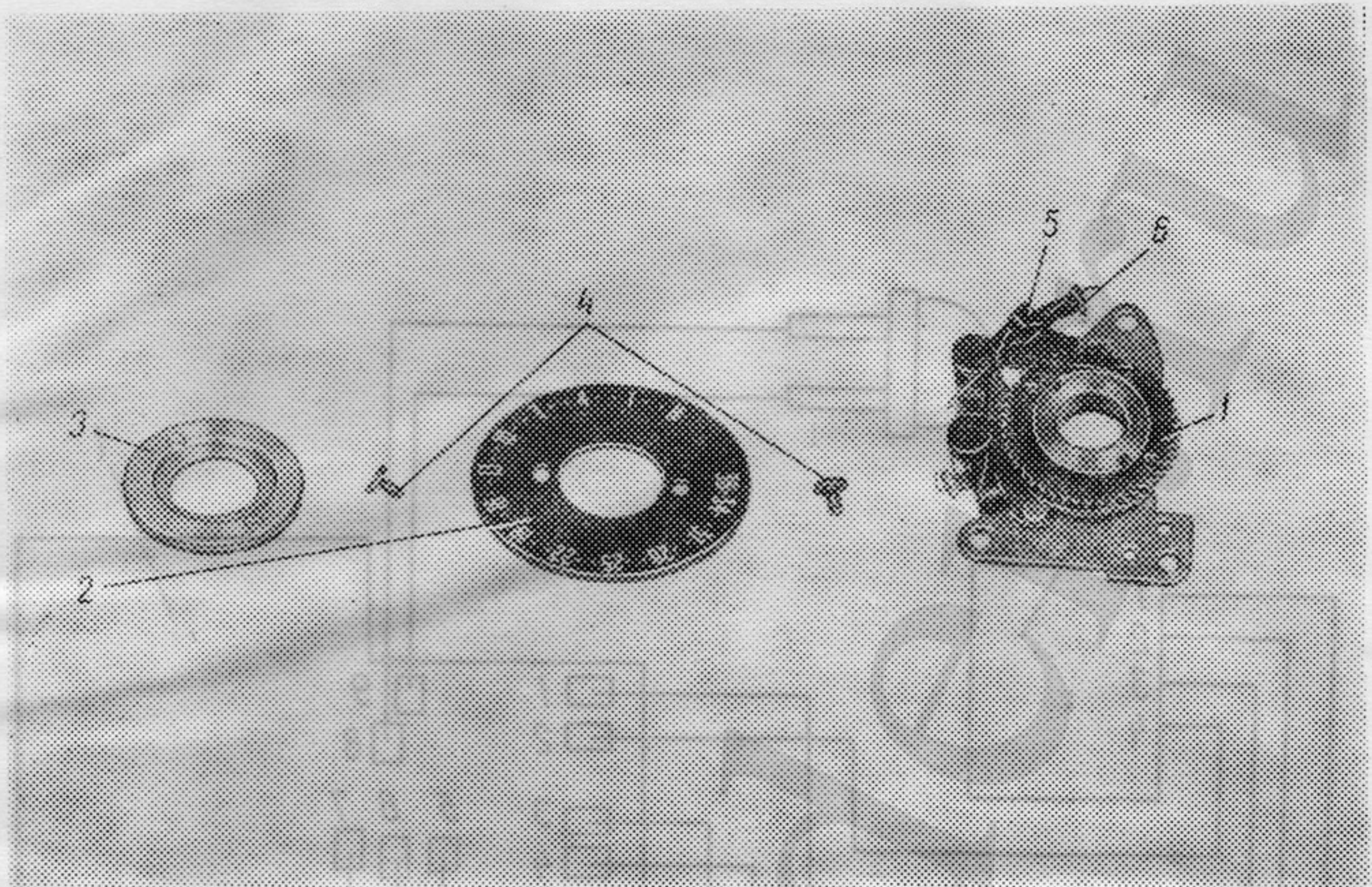
1—колесо храповое 8.364.030; 2—шкала 7.021.456; 3—шайба 9.440.250; 4—винт 8.900.665; 5—собачка 8.364.436; 6—собачка 8.364.435.
