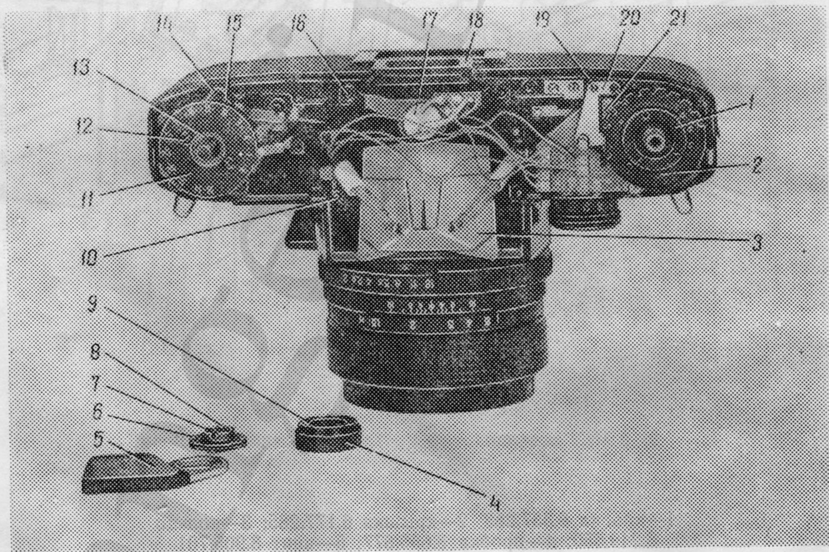
1—гайка 9.438.306; 2—втулка 6.240.156 (потенциометра); 3—видоискатель 5.810.021; 4—кольцо 7.854.650; 5—рычаг 6.354.480; 6—шарик 1.558-60±10 ГОСТ 3722-81; 7—втулка 6.240.139; 8—ролик 8.206.005; 9—втулка 8.229.519; 10—гайка М1,6.6Н.6А.05 ГОСТ 5927-70; 11—шкала 7.021.456; 12—винт 8.900.665; 13—прокладка 8.681.884; 14, 16—винт 8.909.424; 15—счетчик кадров 5.822.188; 17—фоторезистор 5.641.039; 18—окуляр 5.923.244; 19—винт 8.909.424; 20—пружина 8.387.742; 21—плата 6.121.501
