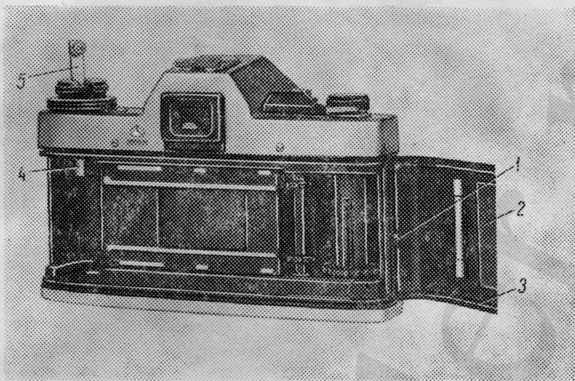
1—винт 8.900.008; 2—пластина 6.462.103; 3—крышка 5.822.146; 4—вилка 8.347.061; 5—рукоятка 6.354.357
