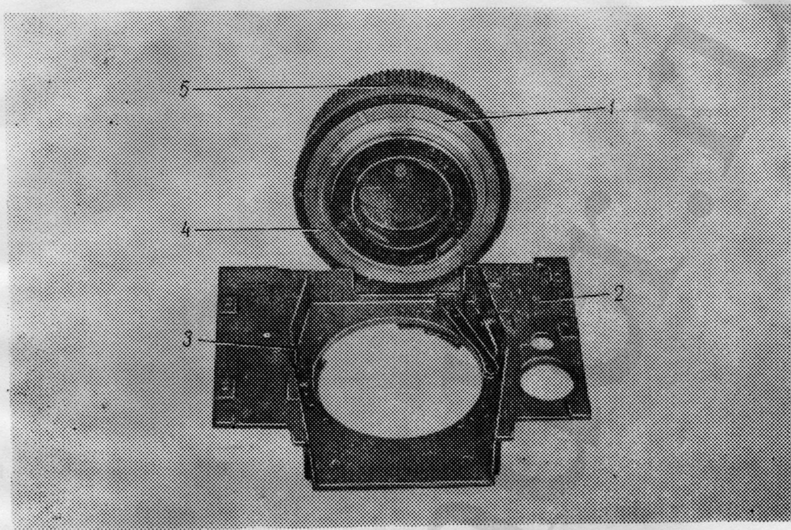
1—байонет 8.127.510; 2—корпус 6.118.038; 3—рычаг 6.354.650; 4—винт 8.903.338-01; 5—объектив 3.873.092.
