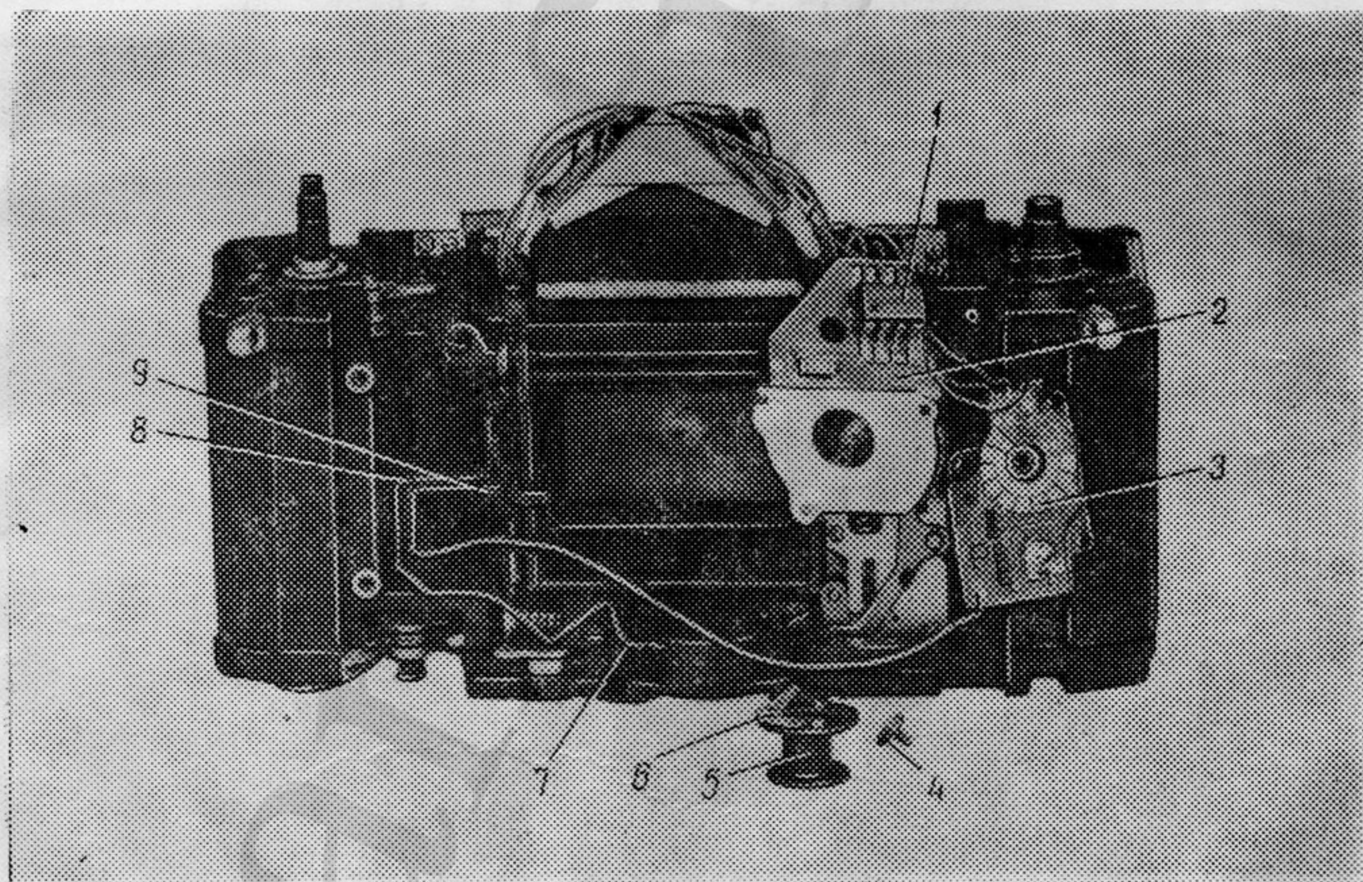
1—микросхема Кр112 ПП2 бко.348.619 ТУ 6231265001 вр; 2—микросборка 5.108.232; 3—микросборка 5.108.233; 4—винт 8.900.029; 5—втулка 9.120.674 (потенциометра); 6—пружина контактная 6.620.272; 7—провод 7.760.132-10; 8—контакт 6.622.368; 9—рычаг 6.354.645
