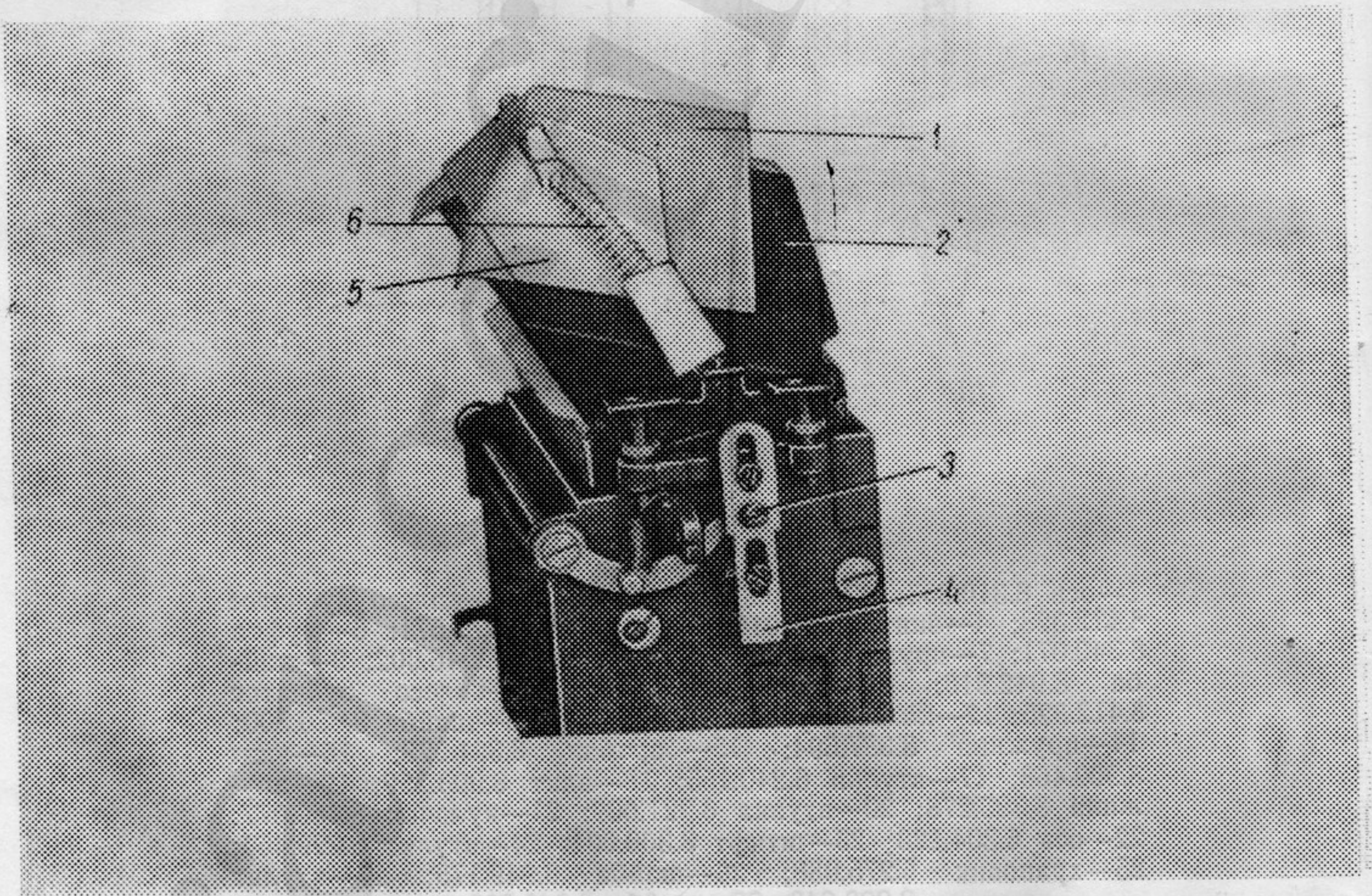
1—прокладка 8.685.541; 2—призма 7.201.184; 3—эксцентрик 8.360.687; 4—рычаг 8.332.593; 5—накладка 8.604.616; 6—пружина 8.380.105
