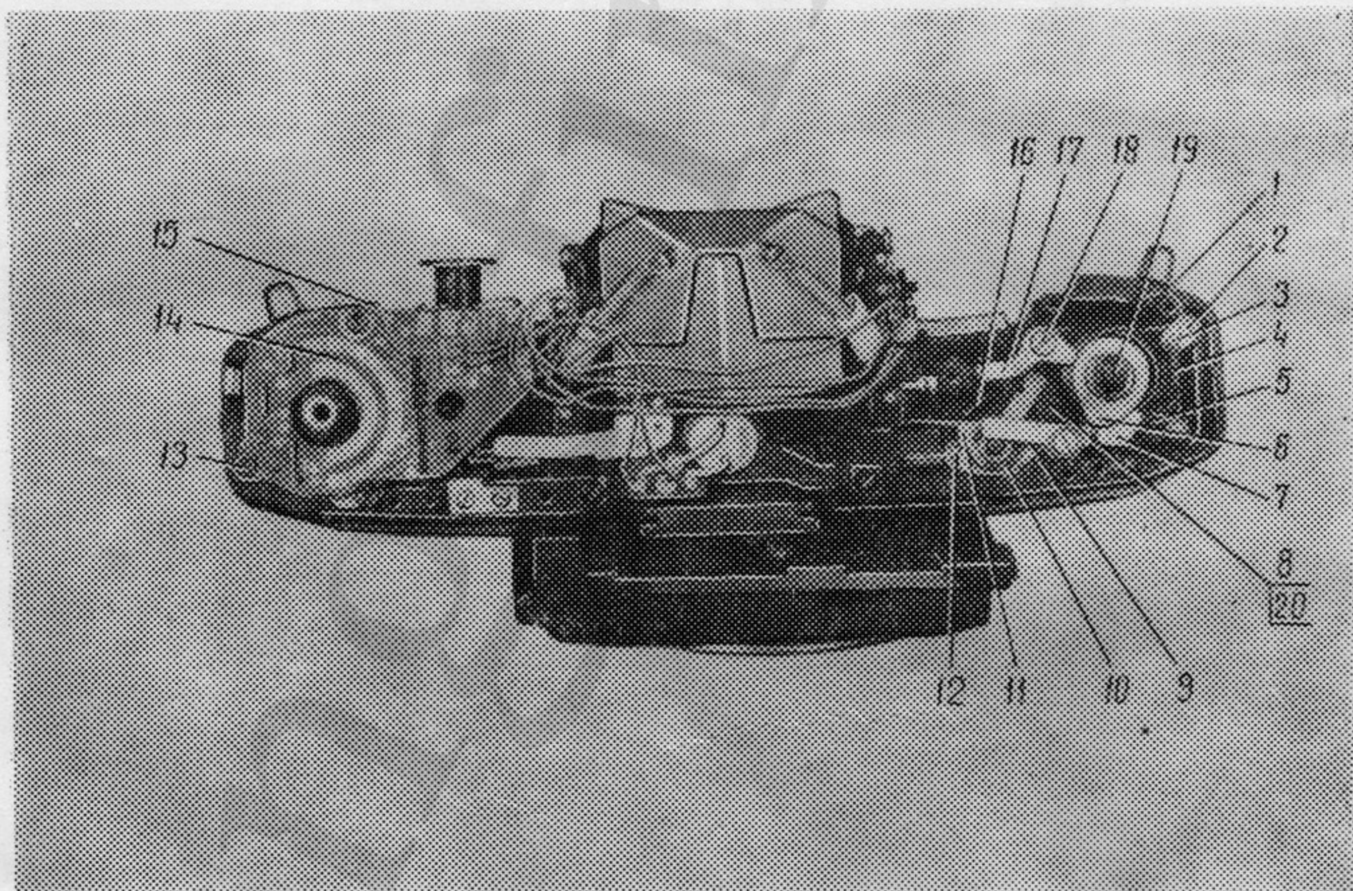
1—пружина 8.385.278; 2—винт 8.900.007; 3—рычаг 6.354.315; 4—пружина 8.380.042; 5—рычаг 8.332.504; 6—кулачок 8.360.077; 7—рычаг 6.354.402; 8—втулка 6.240.155; 9—фланец 8.231.039; 10—шайба 8.946.022; 11—рычаг 8.332.502; 12—винт 8.903.060; 13—винт 8.909.424; 14—микросборка 5.108.232; 15—лакоткань; 16—пружина 8.385.184-01; 17—рычаг 6.354.386; 18—винт 8.900.013; 19—ось 6.304.123; 20—винт 8.903.080
