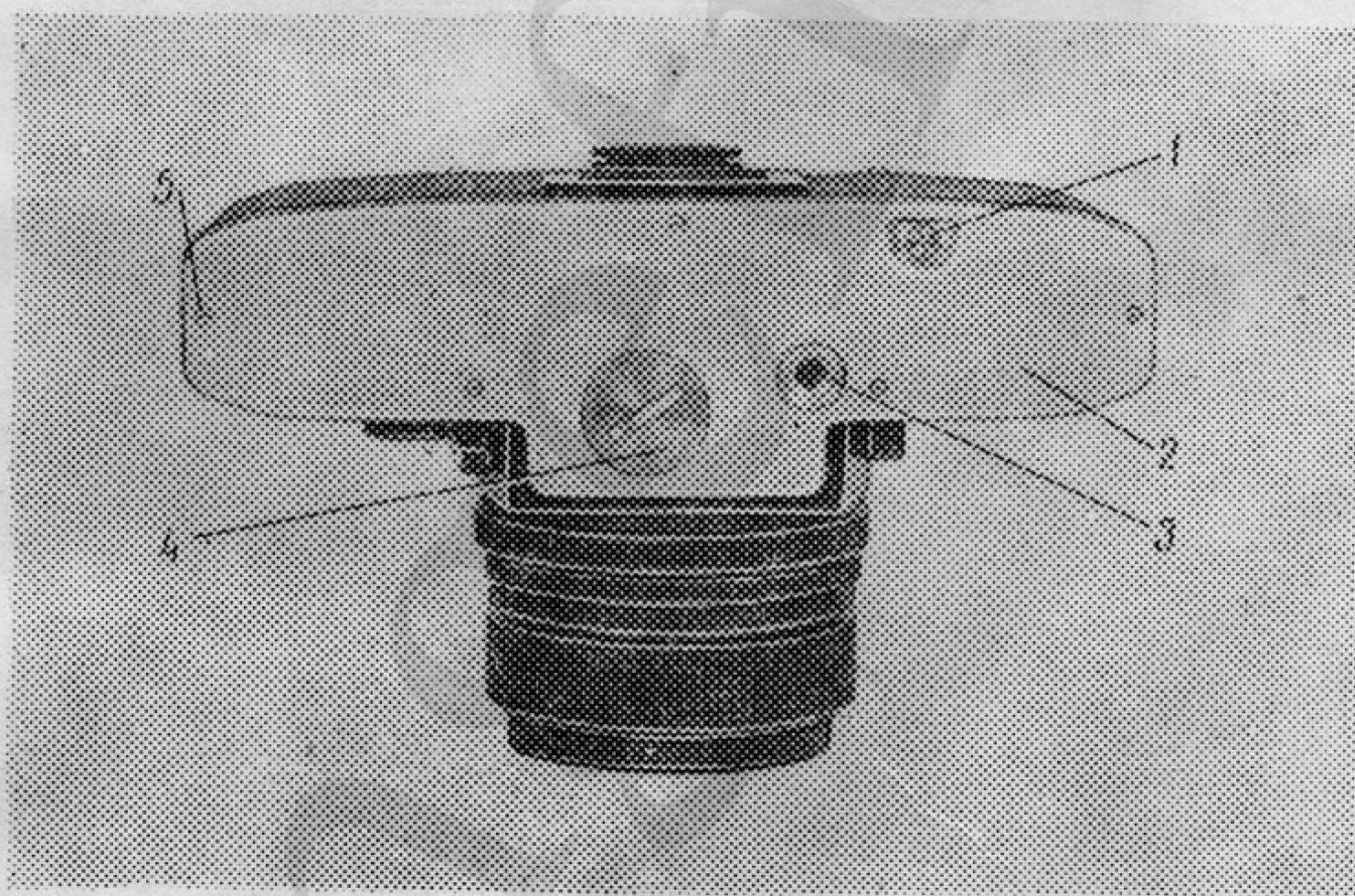
1—кнопка 8.337.283; 2—крышка 6.177.285; 3—кольцо 8.249.550; 4—пробка 8.656.677; 5—винт 8.905.761
