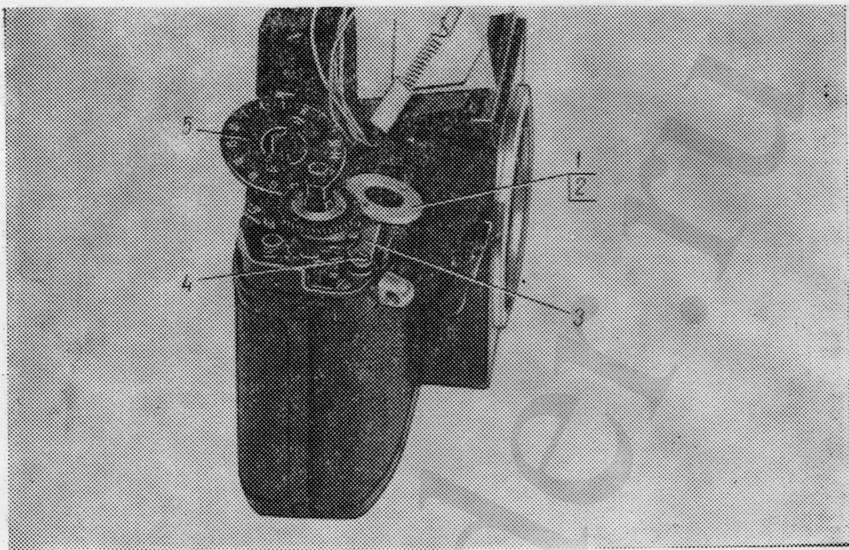
1—шайба 9.440.250; 2—шайба 9.440.257; 3—счетчик кадров 5.822.188; 4—винт 8.909.424; 5—шкала 7.021.456
