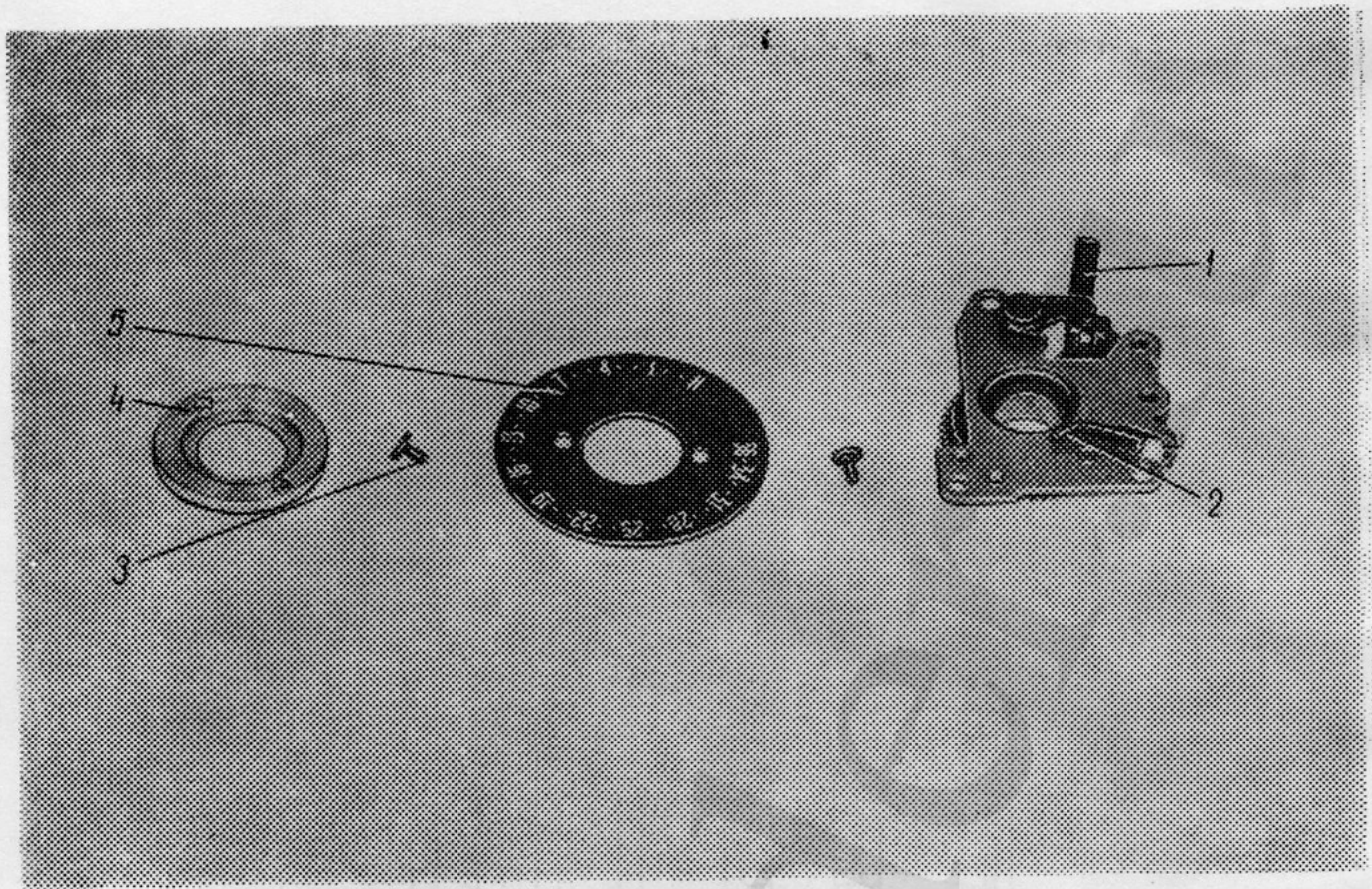
1—рычаг 8.332.572; 2—рычаг 8.332.516; 3—винт 8.900.665; 4—шайба 9.440.250; 5—шкала 7.021.456
