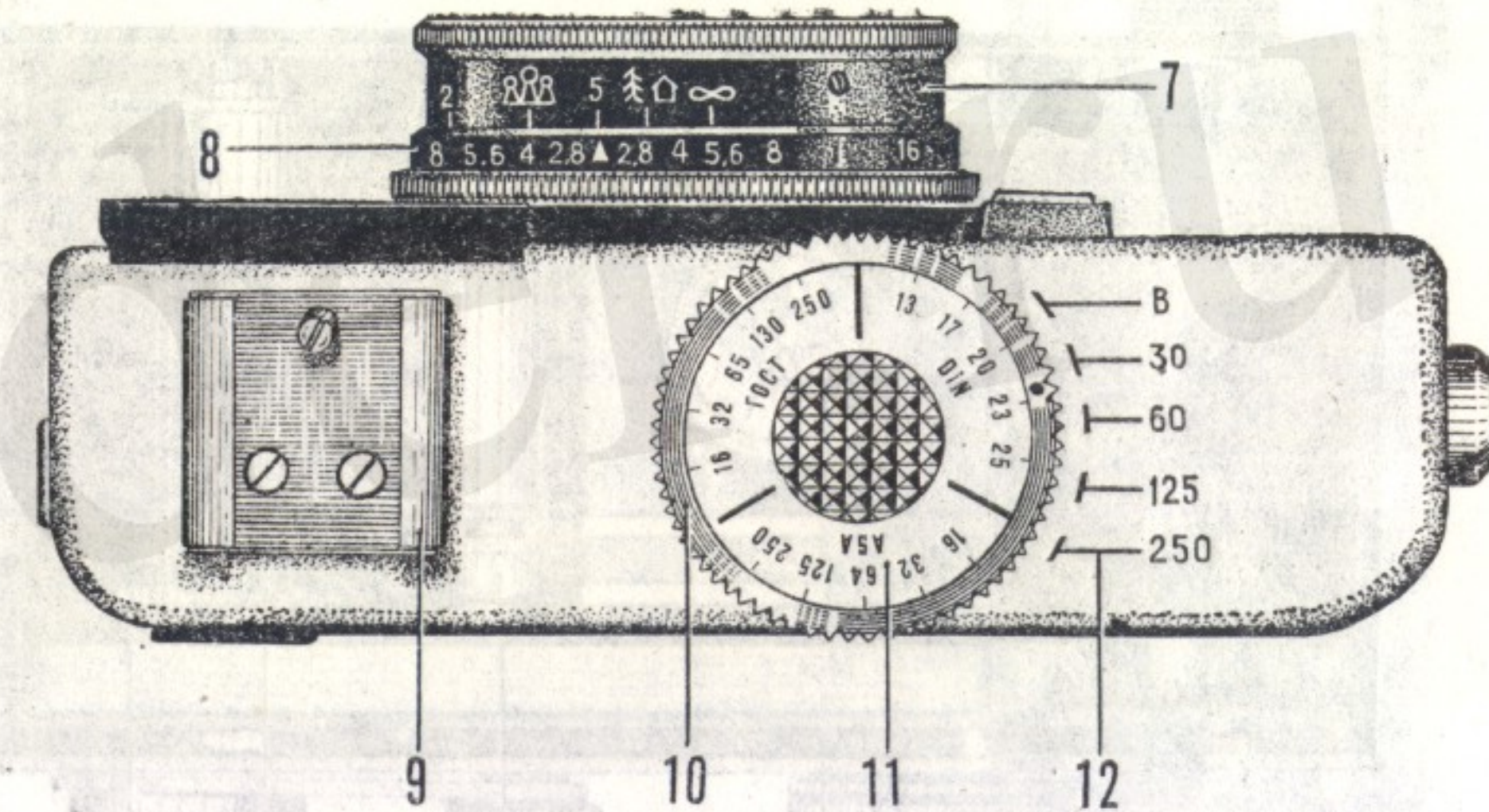
Рис. 2. Вид сверху.
