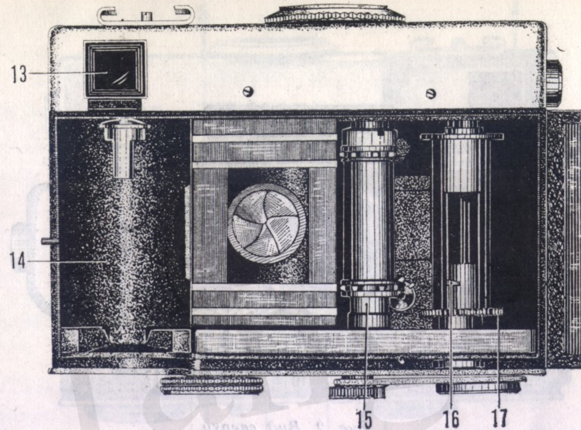
Рис. 3. Фотоаппарат с открытой задней крышкой
