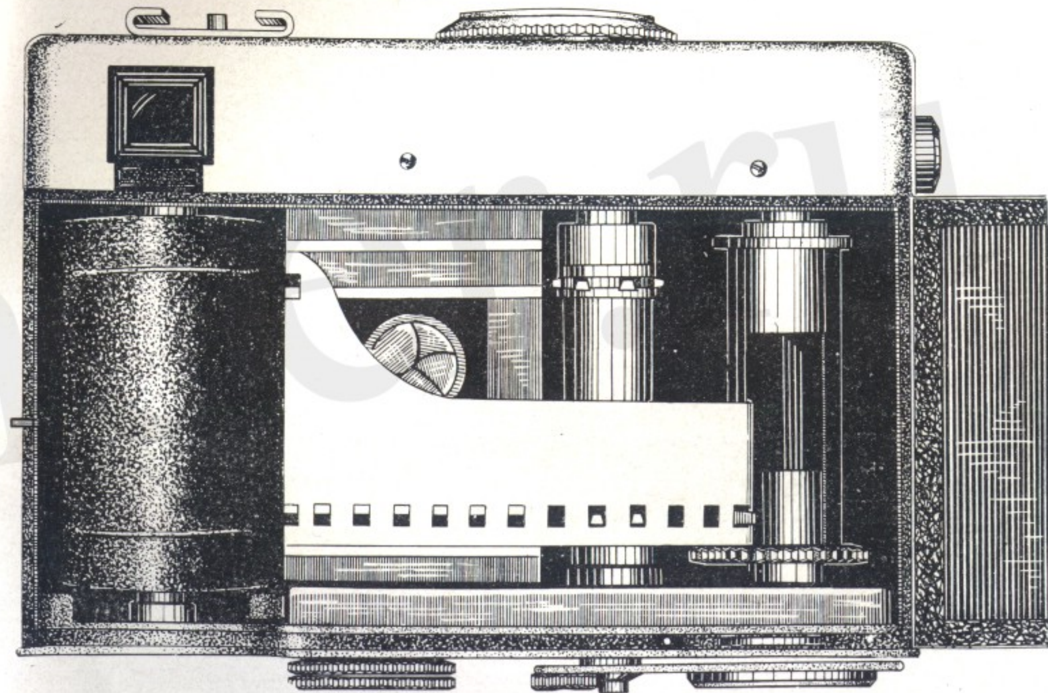
Рис. 8. Фотоаппарат с заряженной кассетой.
