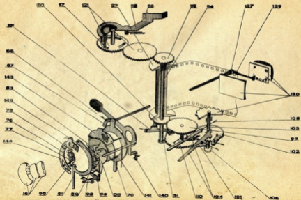
Кинематическая схема фотоаппарата «Вьюга»
