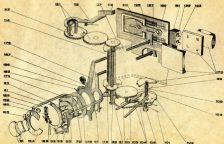
Кинематическая схема фотоаппарата «Силуэт-электрон»
