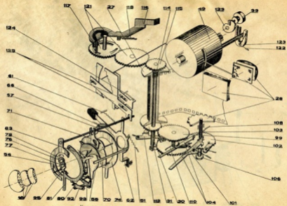
Кинематическая схема фотоаппарата «Вилна-авто»
