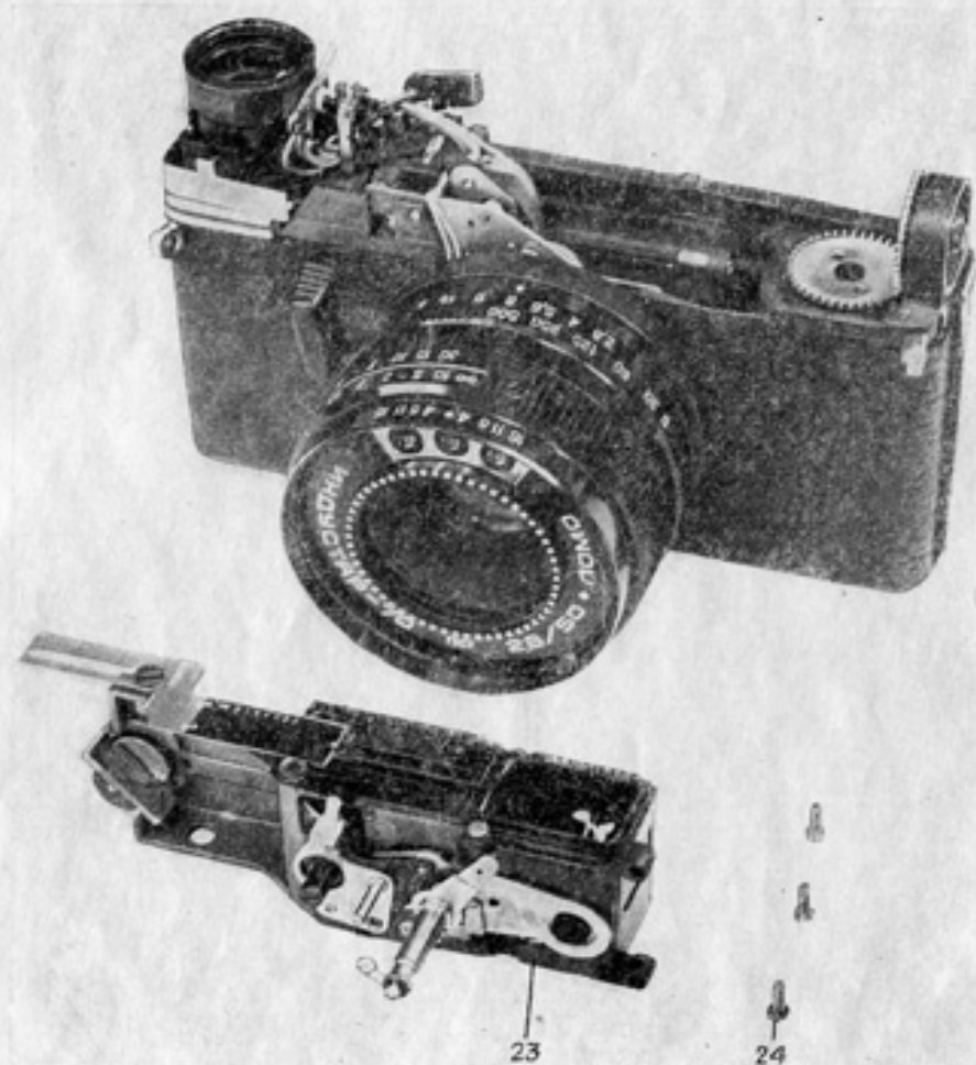
Рис. 5. Фотоаппарат со снятым дальномером 23
