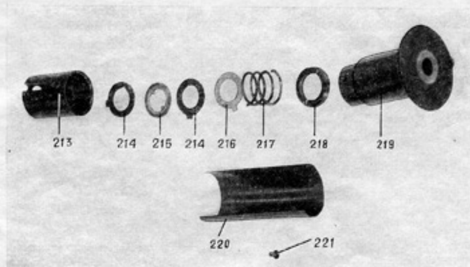
Рис. 21. Детали барабана
