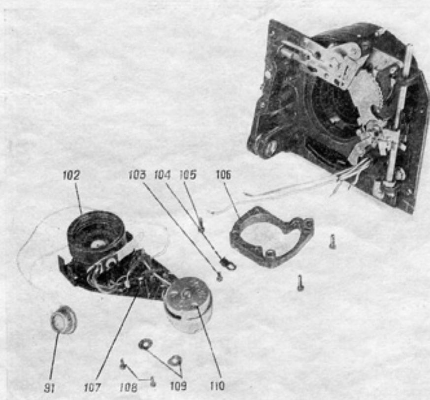
Рис. 10. Сборки и детали платы с затвором 29
