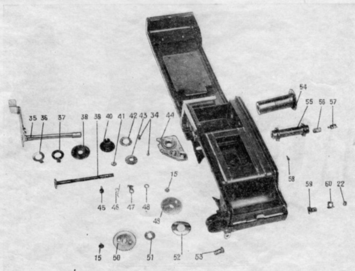
Рис. 7. Сборки и детали корпуса
