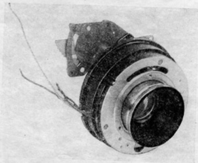
Рис. 13. Затвор 134 с суммирующим механизмом 130 и объективом
