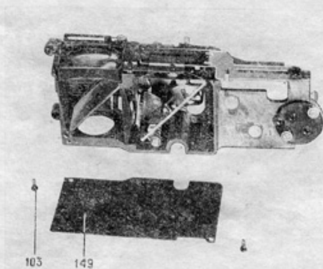
Рис. 14. Дальномер 23 со снятой крышкой 149
