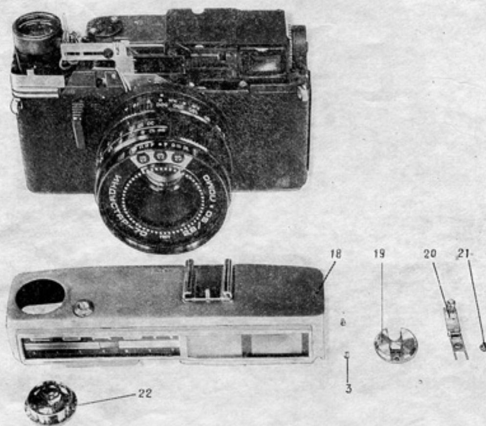
Рис. 4. Фотоаппарат со снятой верхней крышкой 18
