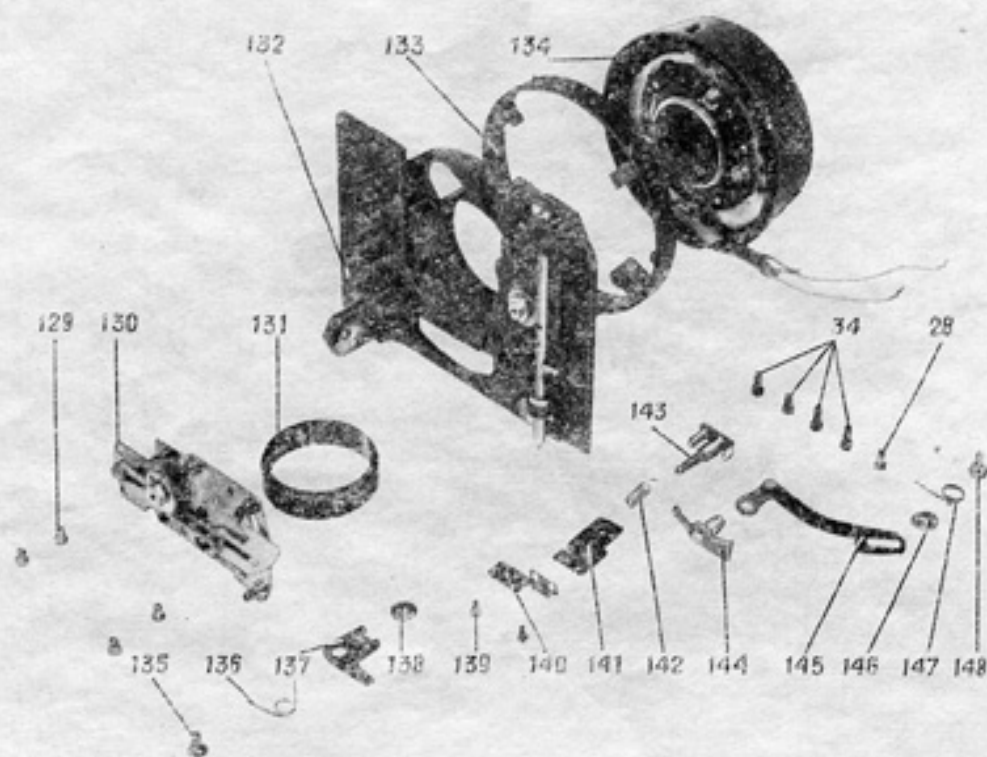
Рис. 12. Сборки и детали платы с затвором 29
