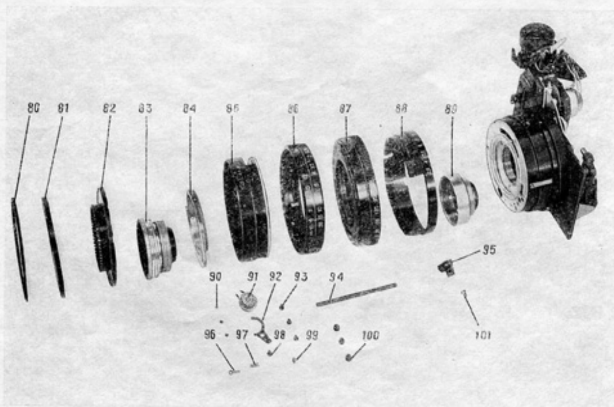
Рис. 9. Сборки и детали платы с затвором 29
