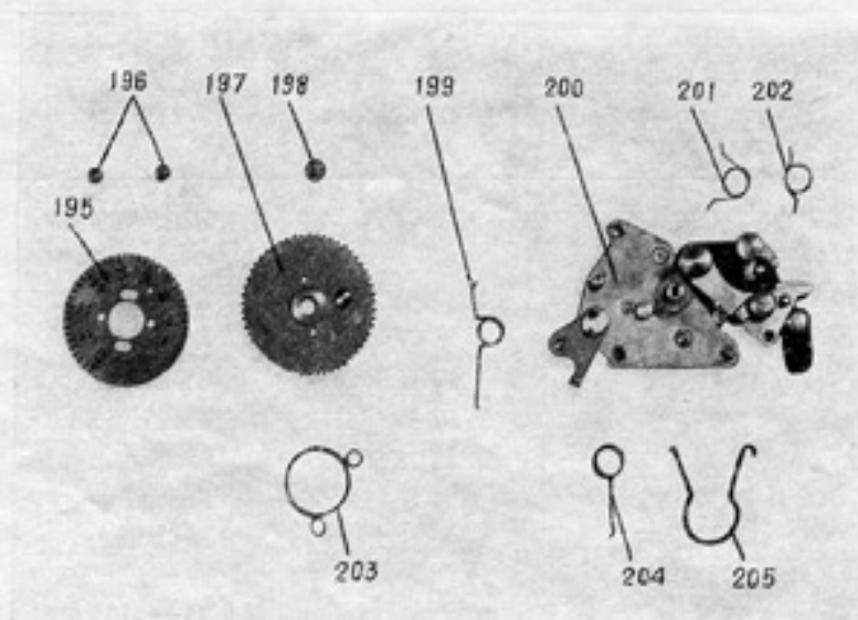
Рис. 19. Сборки и детали счетчика кадров 17
