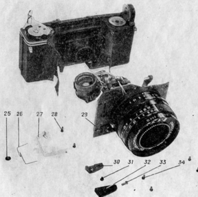
Рис. 6. Фотоаппарат со снятой платой с затвором 29
