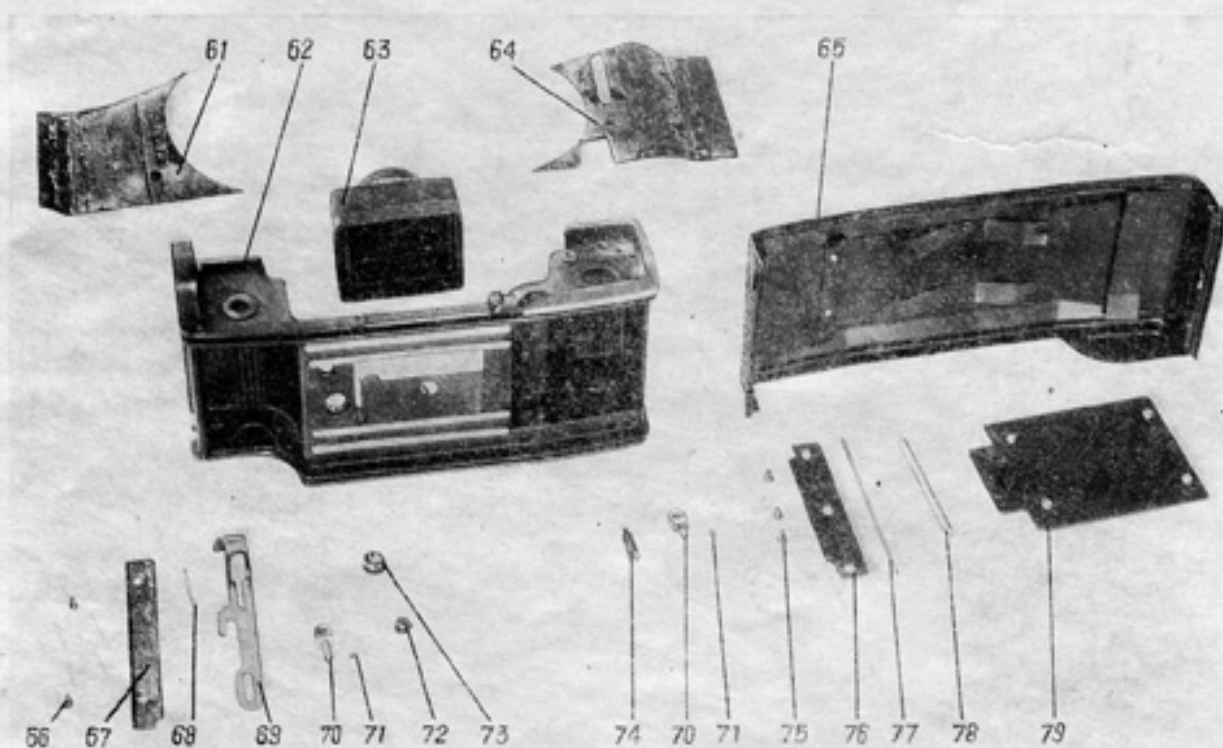
Рис. 8. Сборки и детали корпуса
