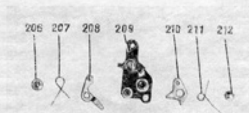
Рис. 20. Сборка и детали платы с рычагами 11
