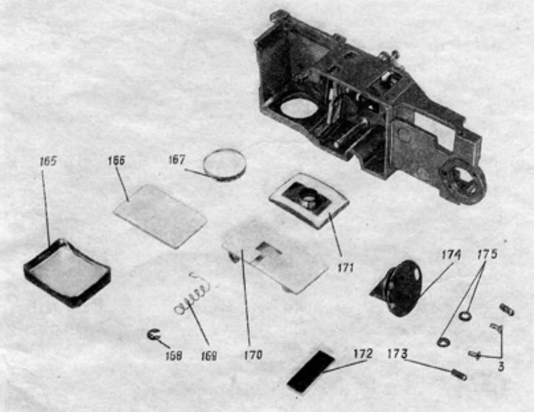
Рис. 16. Сборки и детали дальномера 23
