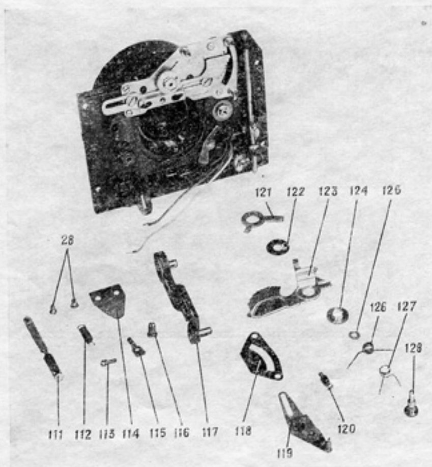
Рис. 11. Сборки и детали платы с затвором 29
