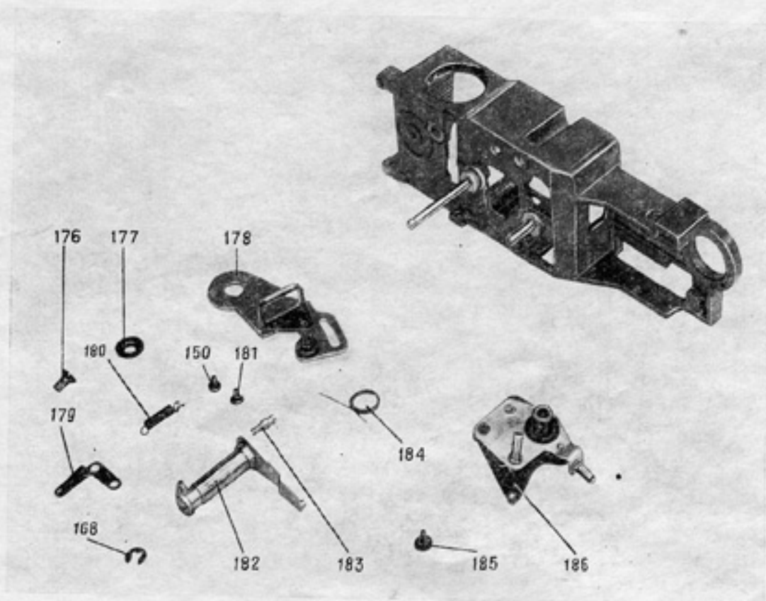
Рис. 17. Сборки и детали дальномера 23
