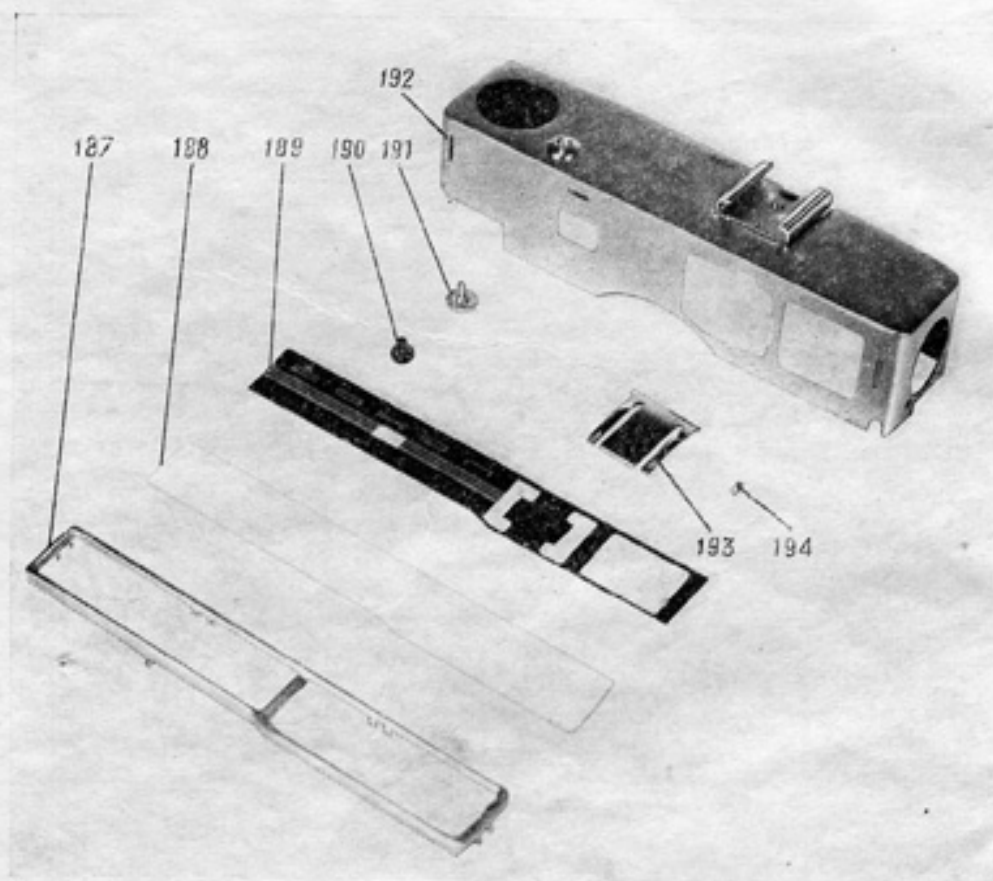
Рис. 18. Сборки и детали верхней крышки 18
