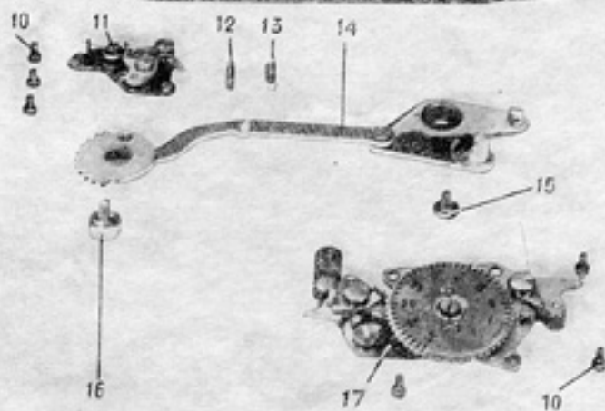
Рис. 3. Фотоаппарат со снятыми счетчиками кадров 17, платой с рычагами блокировки 11 и рычагом взвода затвора 14
