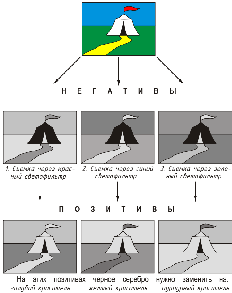
Рис. 24. Схема получения цветоделенных негативов при съемке окрашенных предметов через светофильтры и позитивы, полученные с негативов
