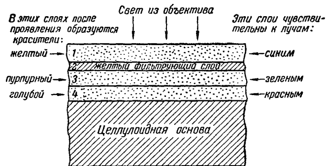
Рис. 26. Схематический разрез многослойной плёнки для цветной фотографии
