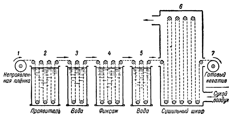
Рис. 8. Схема проявочной машины для киноплёнки
