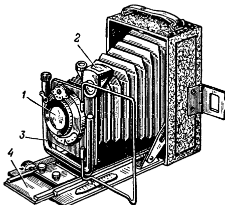
Рис. 22. Общий вид пластиночной камеры „Фотокор“:
