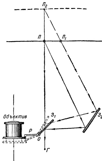
Рис. 15. Схема, поясняющая устройство дальмера для наводки на резкость:
